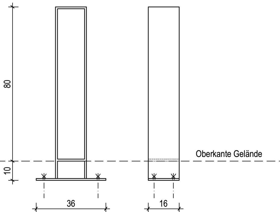
Vorderansicht
