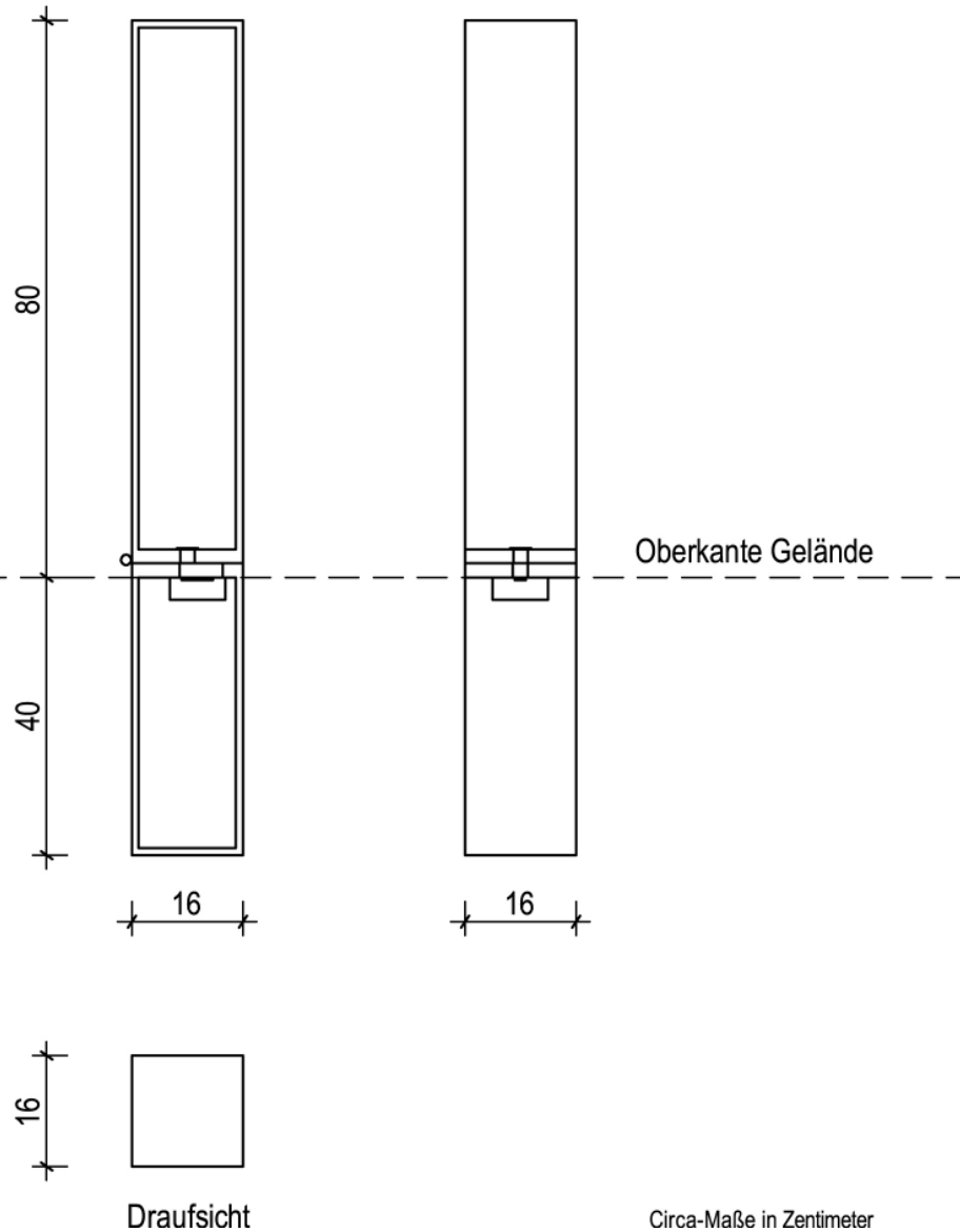
Vorderansicht
